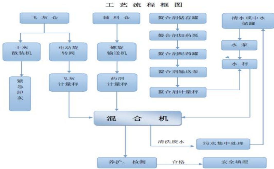
飞灰固化处理流程图
